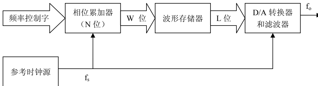
图 1 DDS 的基本原理框图
