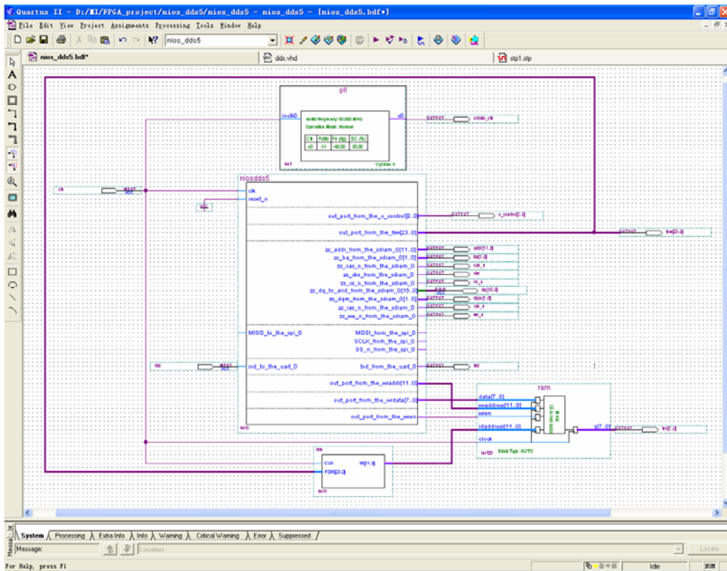
图 5 片上系统顶层设计图
