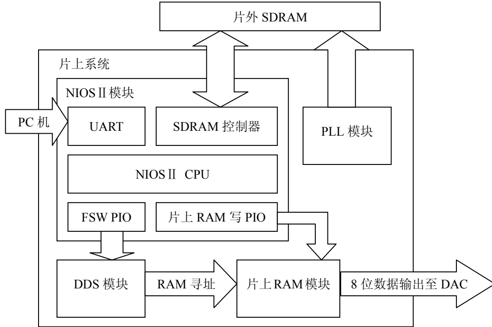
图 4 片上系统框图
